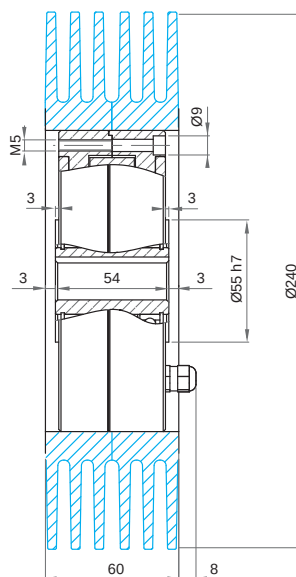
B.351.R freno con radiatore brake with radiator
