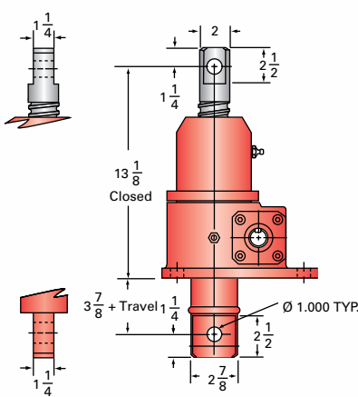
10-BSJ-DC & 10HL-BSJ-DC DOUBLE CLEVIS
