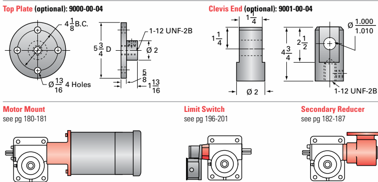
10-BSJ & 10HL-BSJ Options
