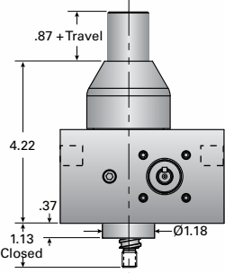
0.5C-BSJ-I &amp; 0.5CHL-BSJ-I INVERTED
