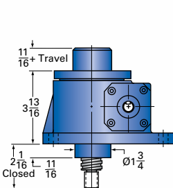
2.5-MSJ-I INVERTED
