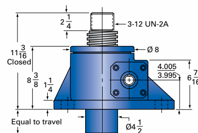
35-MSJ-U UPRIGHT
