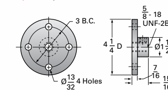
2-BSJ Options
