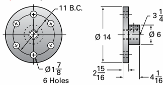
100-BSJ Options
