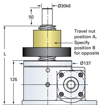
EM10-MSJ-UR UPRIGHT ROTATING
