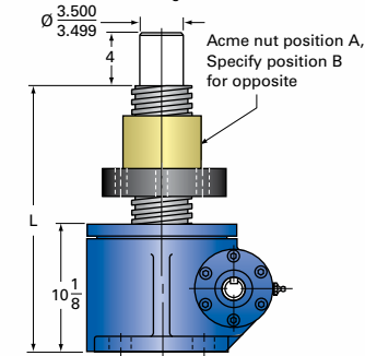
50-MSJ-UR UPRIGHT ROTATING
