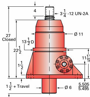
75-BSJ-U UPRIGHT
