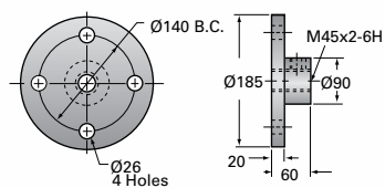
EM20-MSJ Options
