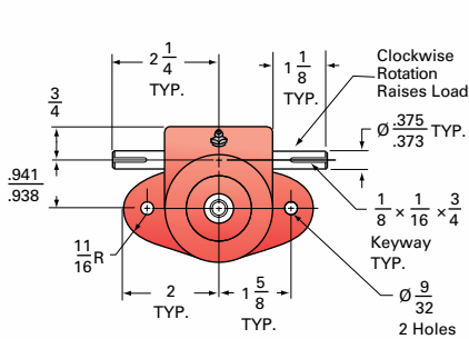
0.5-BSJ & 0.5HL-BSJ TOP VIEW
