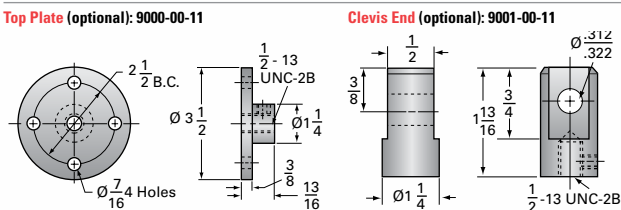
1-MSJ Options
