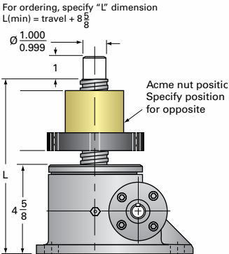
5SS-MSJ-UR UPRIGHT ROTATING
