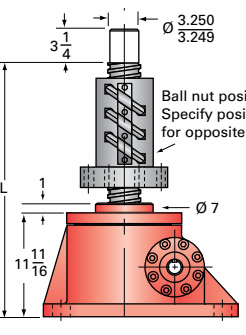
75-BSJ-UR UPRIGHT ROTATING
