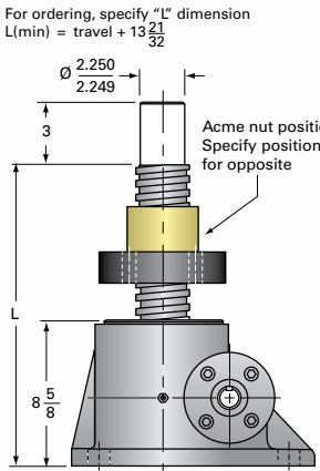
25SS-MSJ-UR UPRIGHT ROTATING
