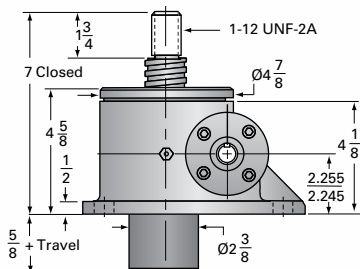
5SS-MSJ-U UPRIGHT
