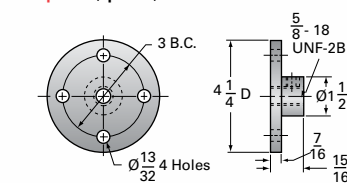
2R-BSJ Options
