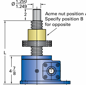
10-MSJ-UR UPRIGHT ROTATING
