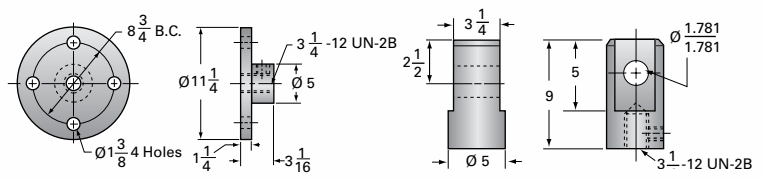
50-BSJ Options
