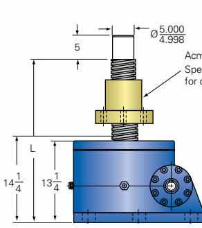
100-MSJ-UR UPRIGHT ROTATING
