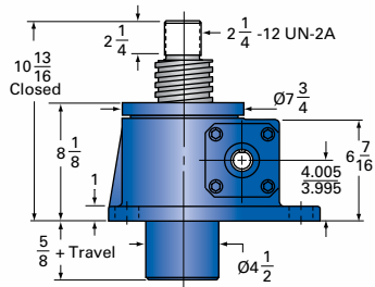
30-MSJ-U UPRIGHT
