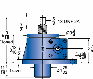
2.5-MSJ-U UPRIGHT
