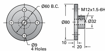
EM1-MSJ Options
