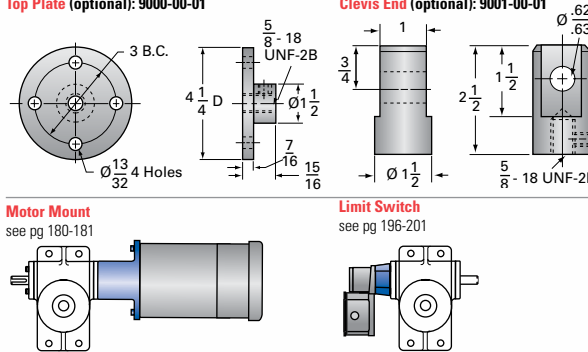
2R-MSJ Options
