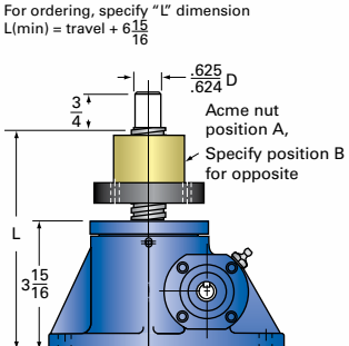
2R-MSJ-UR UPRIGHT ROTATING
