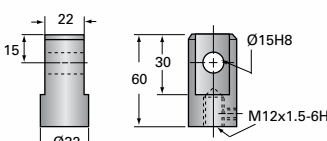
Clevis End (optional): 9001-EM-11
