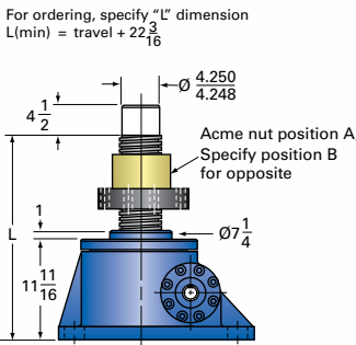
75-MSJ-UR UPRIGHT ROTATING
