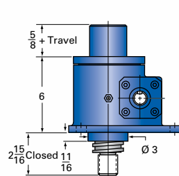
15-MSJ-I INVERTED
