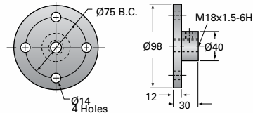
EM2.5-MSJ Options
