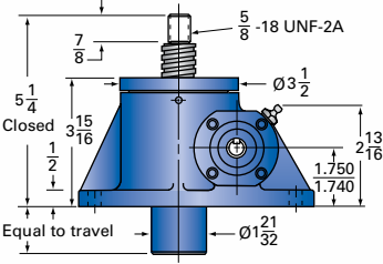
2R-MSJ-U UPRIGHT
