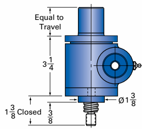
1-MSJ-I INVERTED
