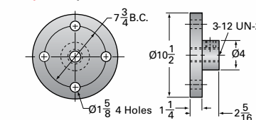
35-MSJ Options
