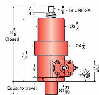
3-BSJ-U UPRIGHT
