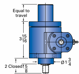
2-MSJ-I INVERTED
