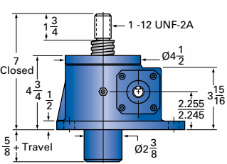
5-MSJ-U UPRIGHT
