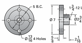
20SS-MSJ Options
