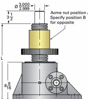
35SS-MSJ-UR UPRIGHT ROTATING
