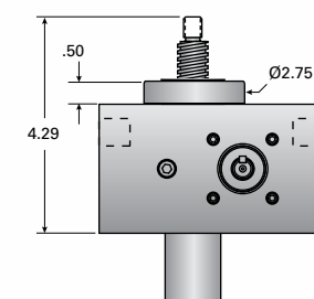
1ABC-MSJ-U UPRIGHT ANTI-BACKLASH
