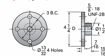
2.5-BSJ Options
