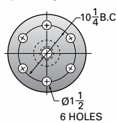
75-BSJ Options
