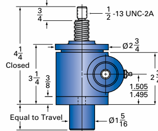
1-MSJ-U UPRIGHT
