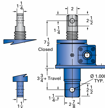
10-MSJ-DC DOUBLE CLEVIS
