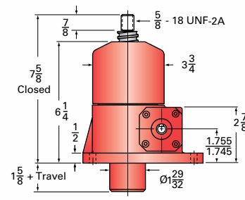
2.5-BSJ-U UPRIGHT
