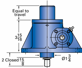
2R-MSJ-I INVERTED
