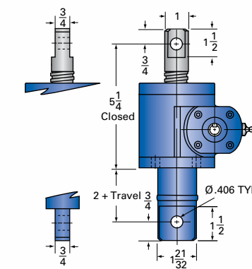
2-MSJ-DC DOUBLE CLEVIS
