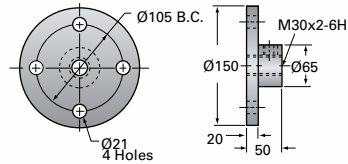
EM10-MSJ Options
