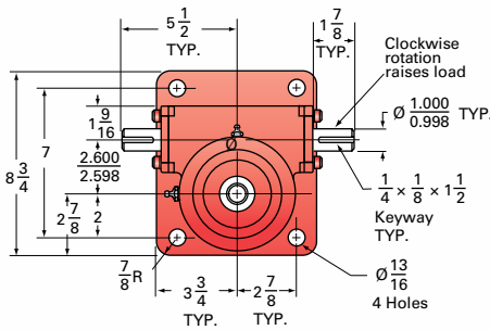
10-BSJ & 10HL-BSJ TOP VIEW
