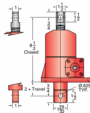
2.5HL-BSJ DOUBLE CLEVIS
