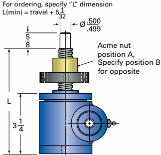
1-MSJ-UR UPRIGHT ROTATING
