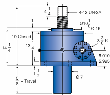
100-MSJ-U UPRIGHT
