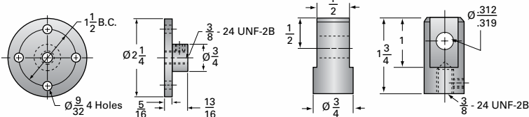
MINI CUBIC JACK Options (Standard Steel Parts)
