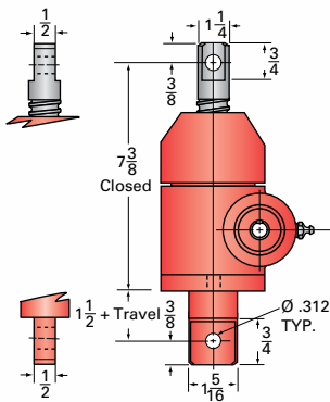
1HL-BSJ-DC DOUBLE CLEVIS
