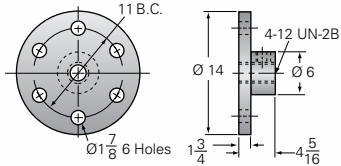
100-MSJ Options
