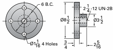
30-MSJ Options
