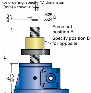
2.5-MSJ-UR UPRIGHT ROTATING
