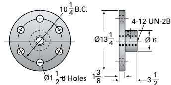
75-MSJ Options
