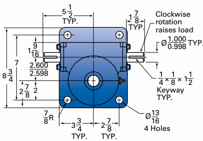
10-MSJ TOP VIEW
