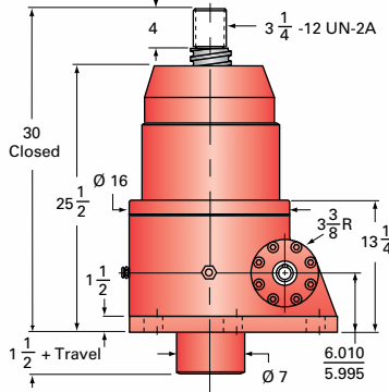
100-BSJ-U UPRIGHT
