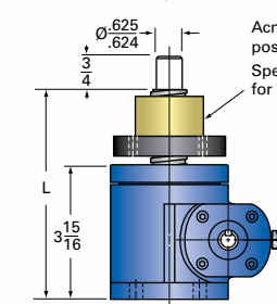
2-MSJ-UR UPRIGHT ROTATING
