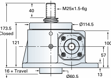
EM5-MSJ-U UPRIGHT
