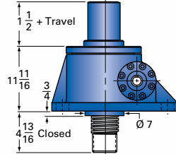
75-MSJ-I INVERTED
