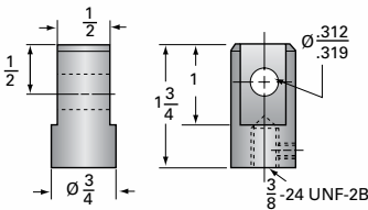
Clevis End (optional): 9001-EM-12
