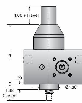
1C-BSJ-I & 1CHL-BSJ-I INVERTED
