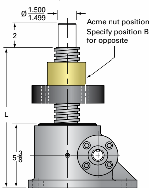
15SS-MSJ-UR UPRIGHT ROTATING
