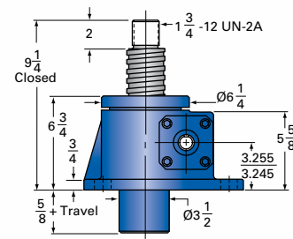
20-MSJ-U UPRIGHT
