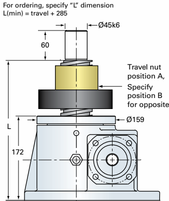
EM20-MSJ-UR UPRIGHT ROTATING
