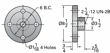
25SS-MSJ Options
