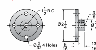
MINI JACK Options
