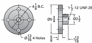
15SS-MSJ Options
