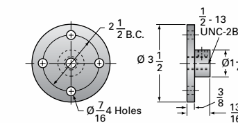
1-BSJ Options
