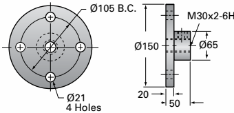
EM10-BSJ Options
