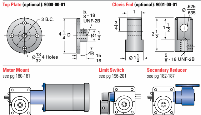
2.5-MSJ Options
