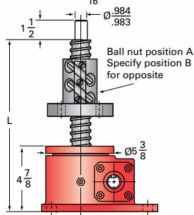
10-BSJ-UR & 10HL-BSJ-UR UPRIGHT ROTATING
