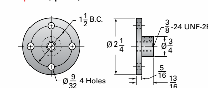
EM05-MSJ Options
