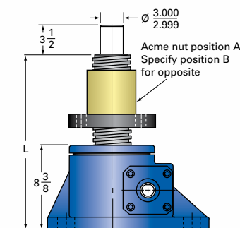
35-MSJ-UR UPRIGHT ROTATING
