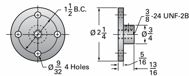
0.5-BSJ & 0.5HL-BSJ Options
