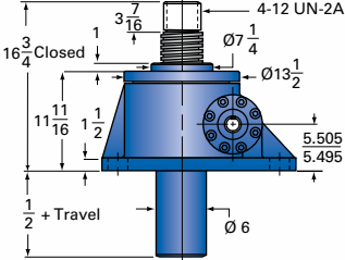
75-MSJ-U UPRIGHT
