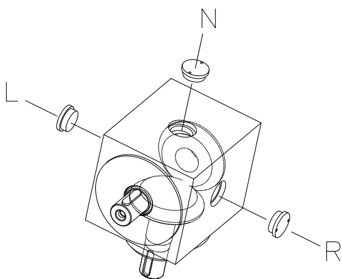
Positionen der Verschlusschrauben positions of the screw plugs
