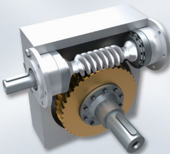
Schneckengetriebe worm gearbox
