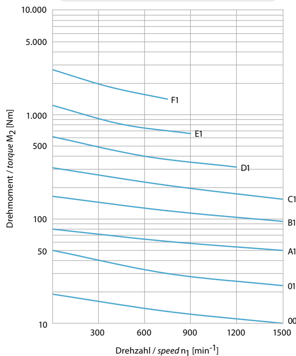
i=n_1:n_2=1:2 (Standard)
