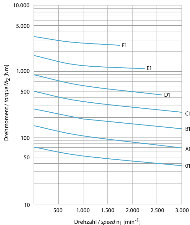
i=n_1:n_2=1:2 (Standard)
