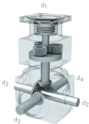
2 zusätzliche Wellenzapfen ZA 2 additional auxiliary shaft extension ZA
